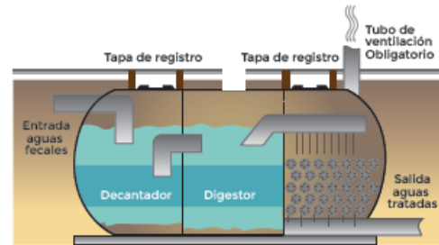
Separador de Fangos
